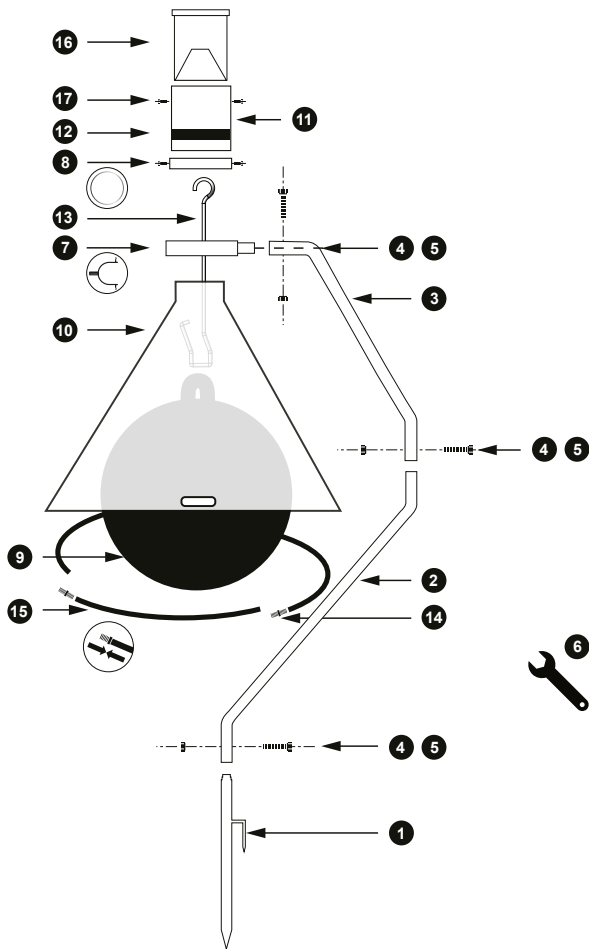
Image 2 : Enfoncer la base du pied dans le sol à l'aide d'un marteau.
