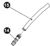
Abb. 3: Verbindung von Verstärkungsschlauch und Schlauchverbindern
