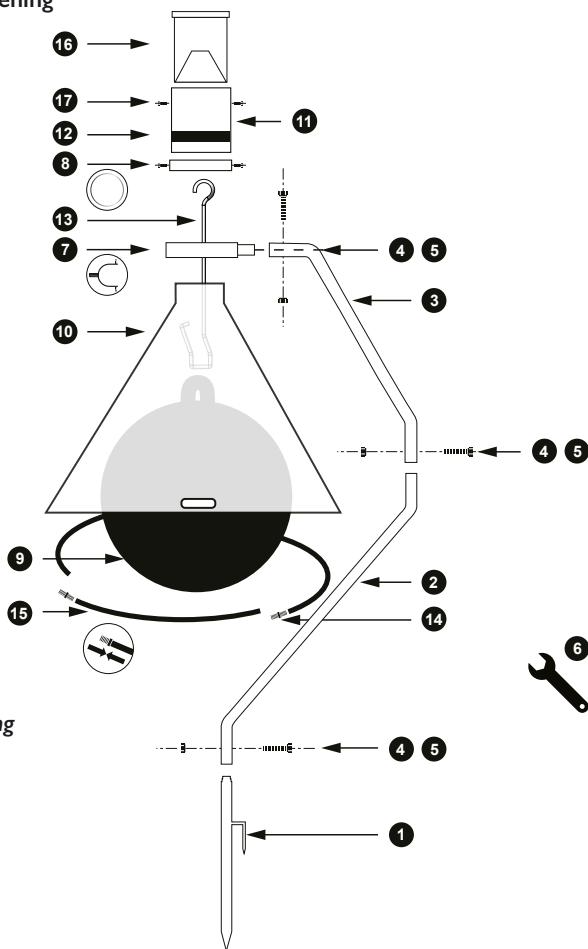
Figuur 3: Montage van de bevestigingsbuis van de kap met het verbindingsstuk.
