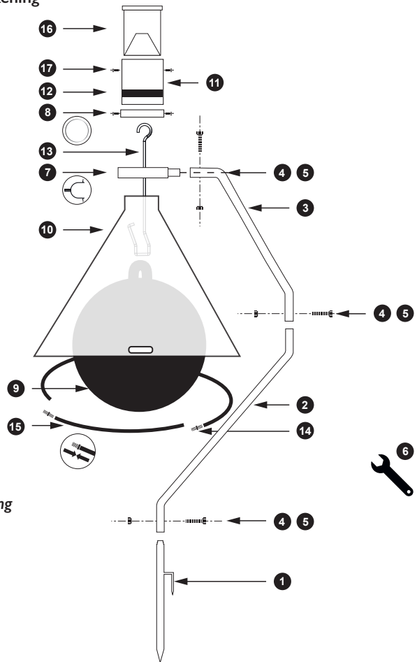
Figuur 3: Montage van de bevestigingsbuis van de kap met het verbindingsstuk.
